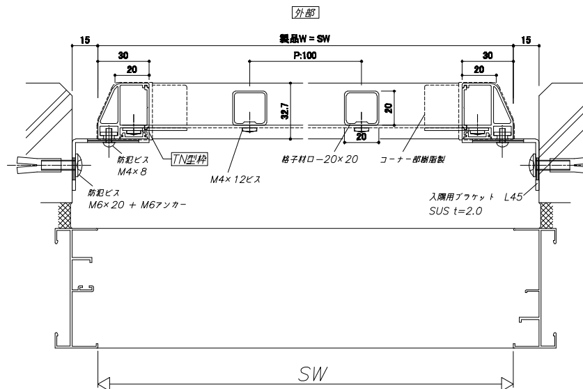
横断面図
