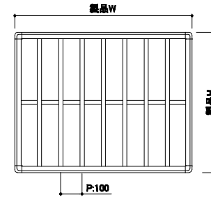
外観姿図
