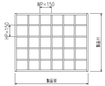
外觀姿図
