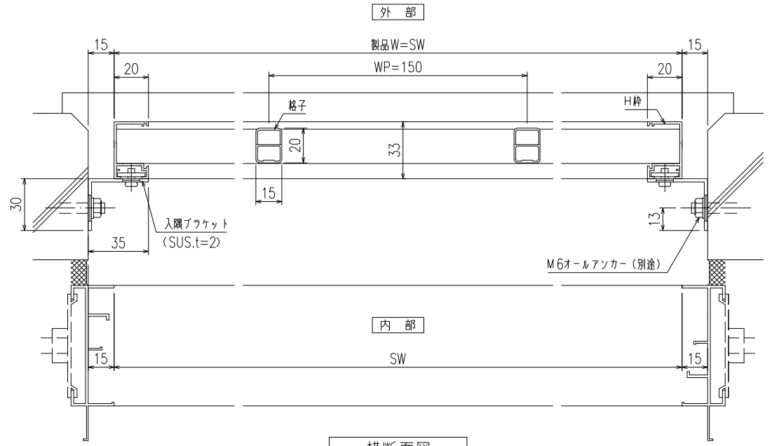
横断面図
