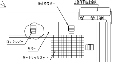
内観詳細図
