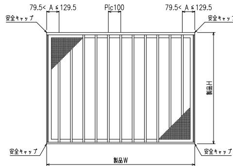
外観姿図
