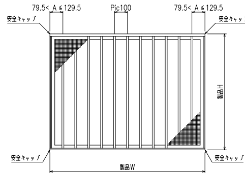
外観姿図
