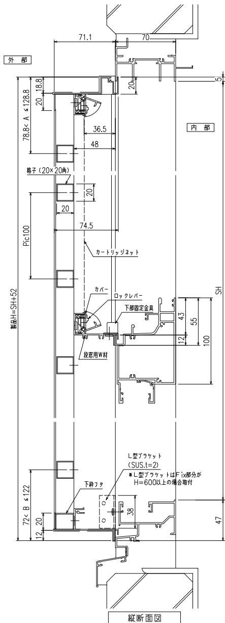
縦断面図
