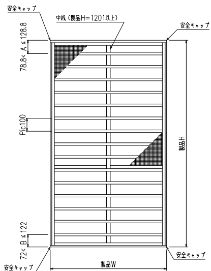
外観姿図
