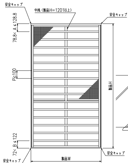
外觀姿図
