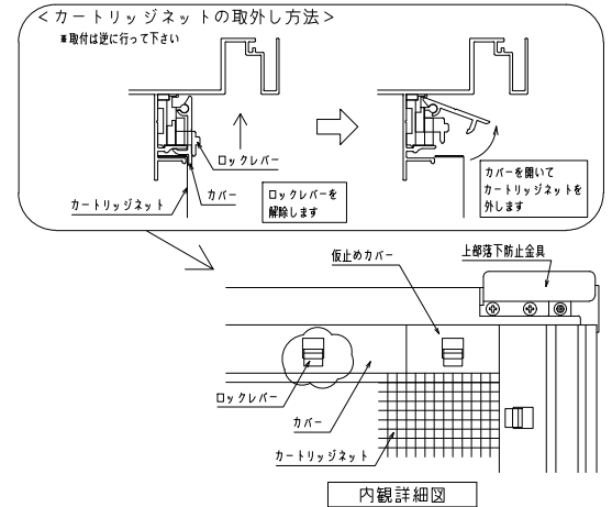
内観詳細図
