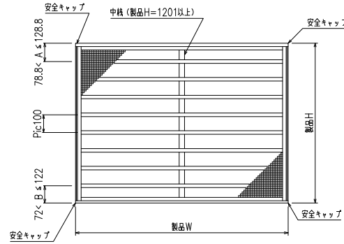
外觀姿図
