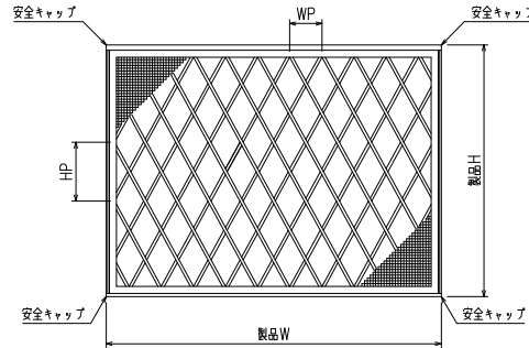
外觀姿図
