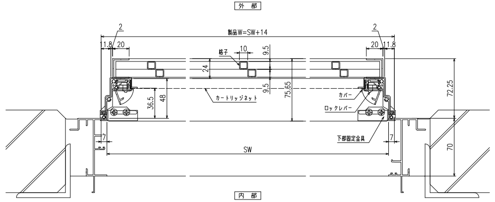
横断面図
