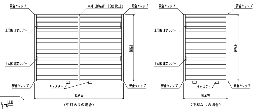
外觀姿図
