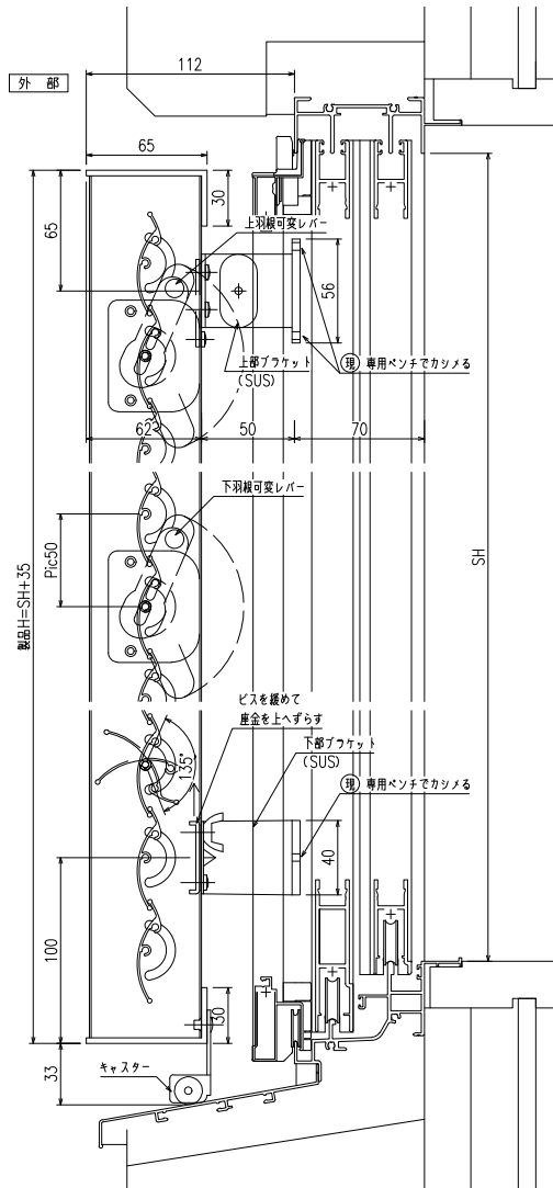
縦断面図
