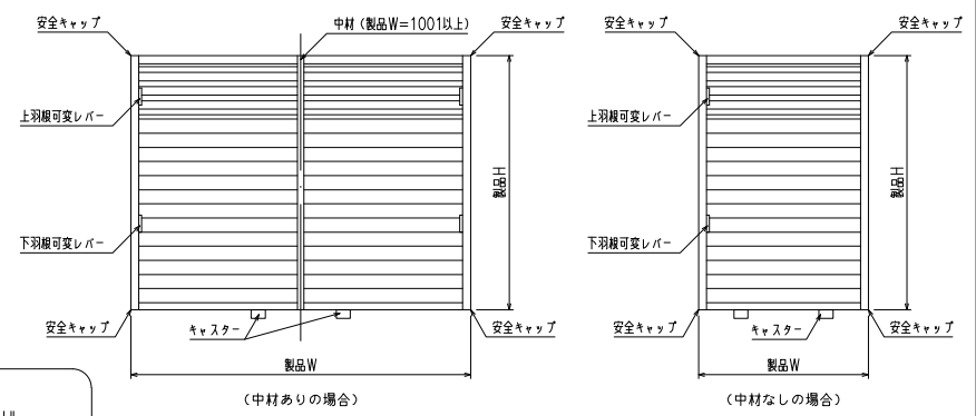
外観姿図
