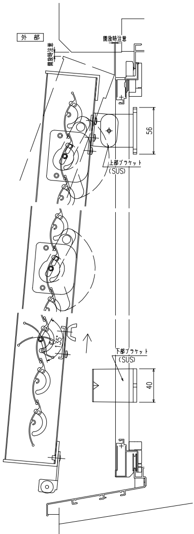
開放詳細図
