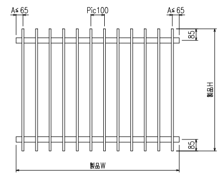
外觀図
