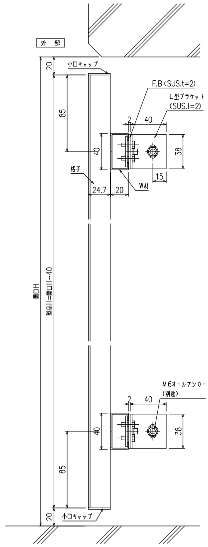
縦断面図
