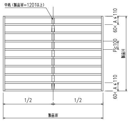
外觀姿図
