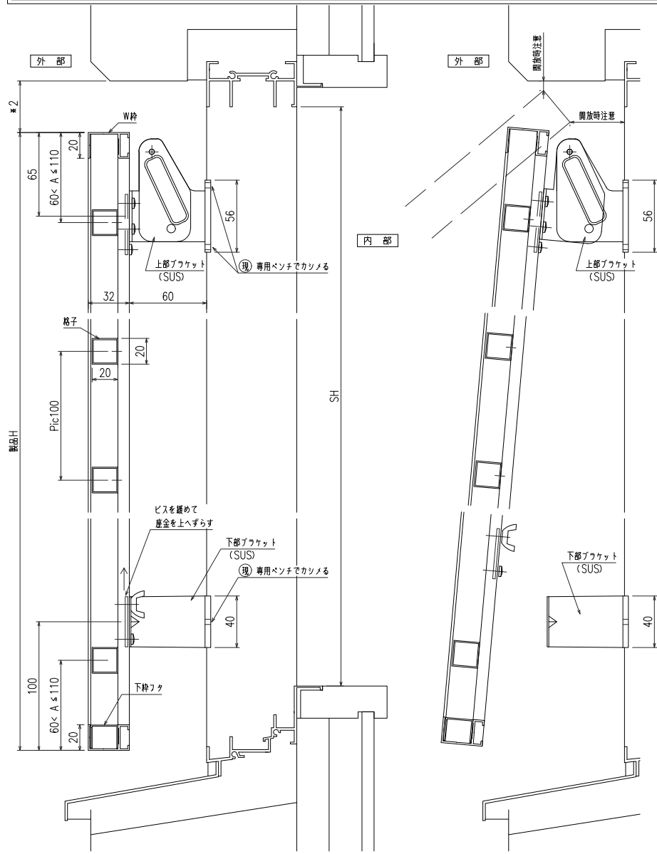
縦断面図
