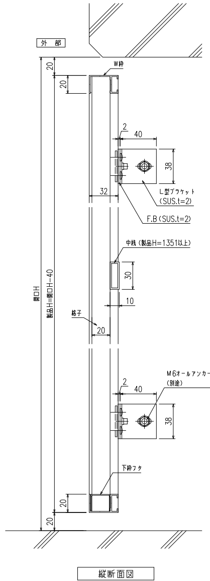
縦断面図
