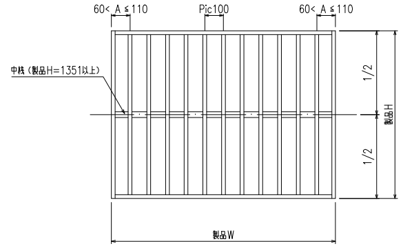
外觀姿図
