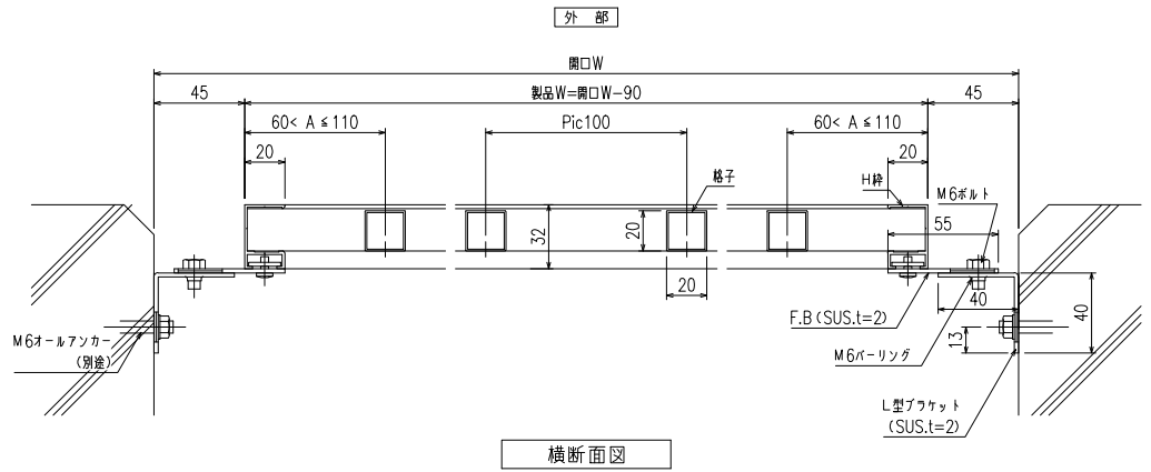
横断面図
