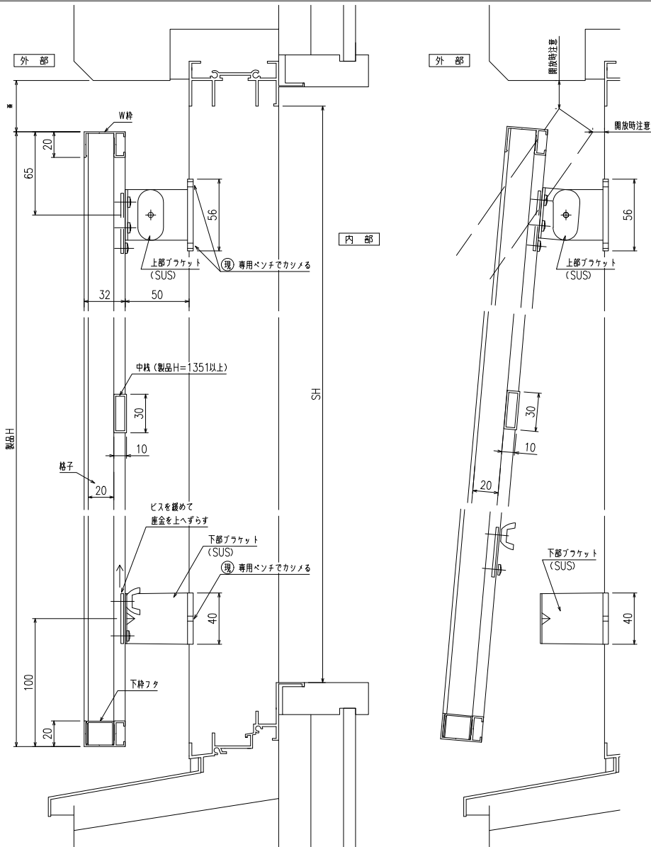
縦断面図
