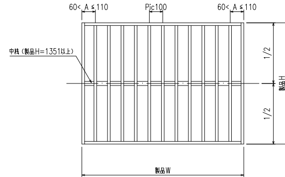
外観姿図
