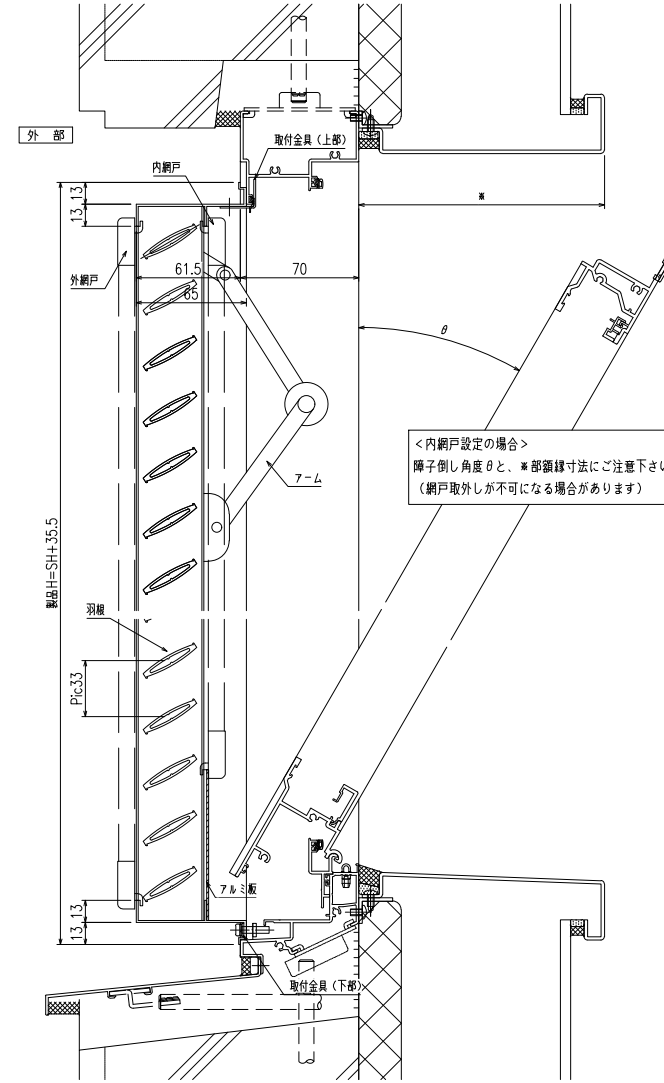
縦断面図
