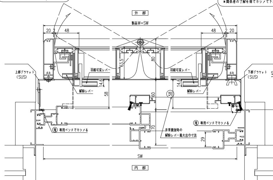
横断面図
