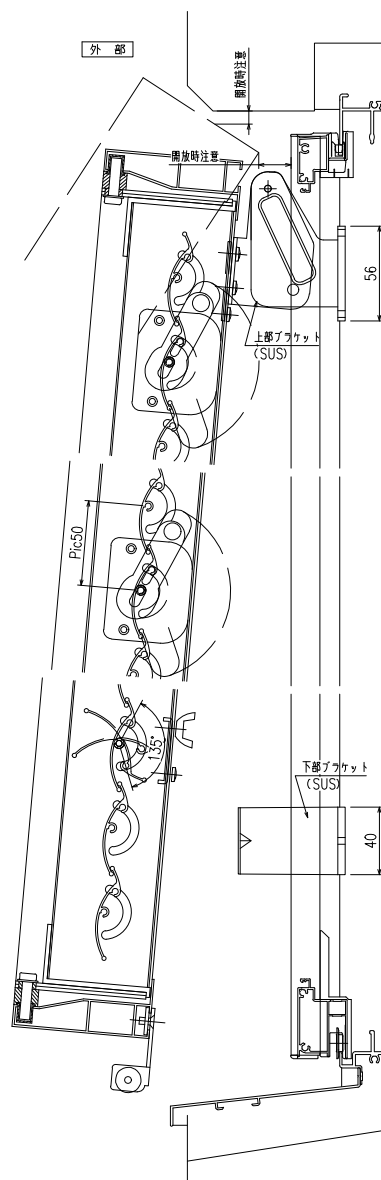
開放詳細図
