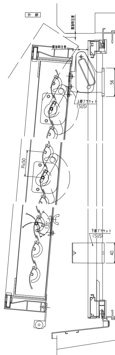
開放詳細図
