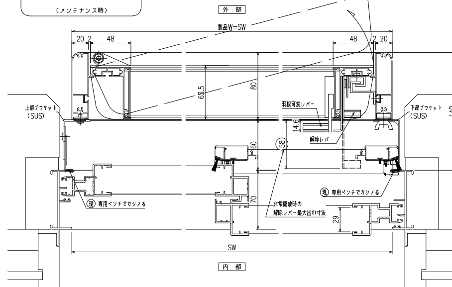
横断面図
