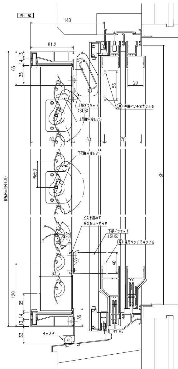
縦断面図
