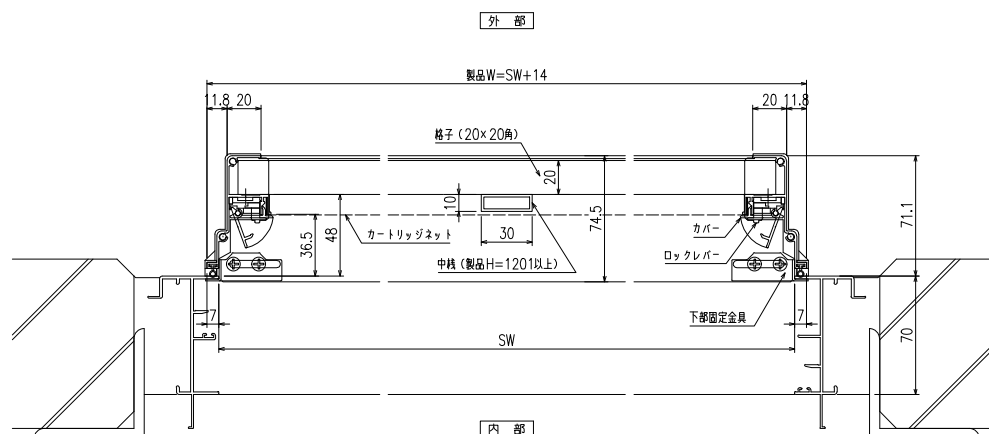
横断面図
