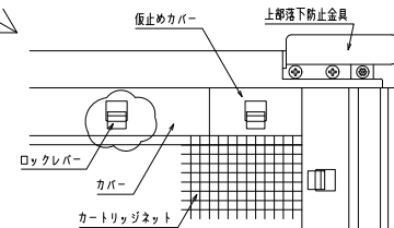
内観詳細図
