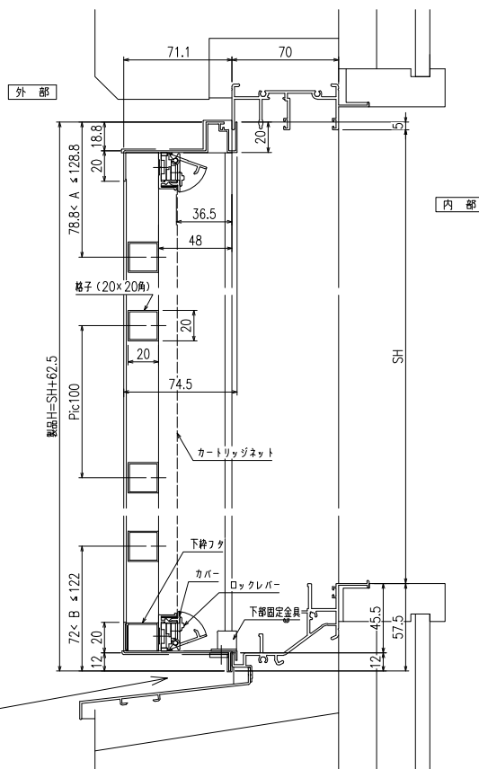
縦断面図
