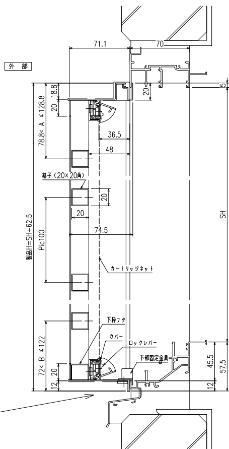
縦断面図
