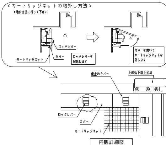
内観詳細図
