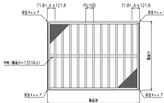
外観姿図
