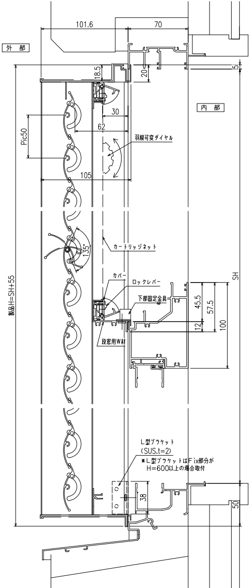
縦断面図
