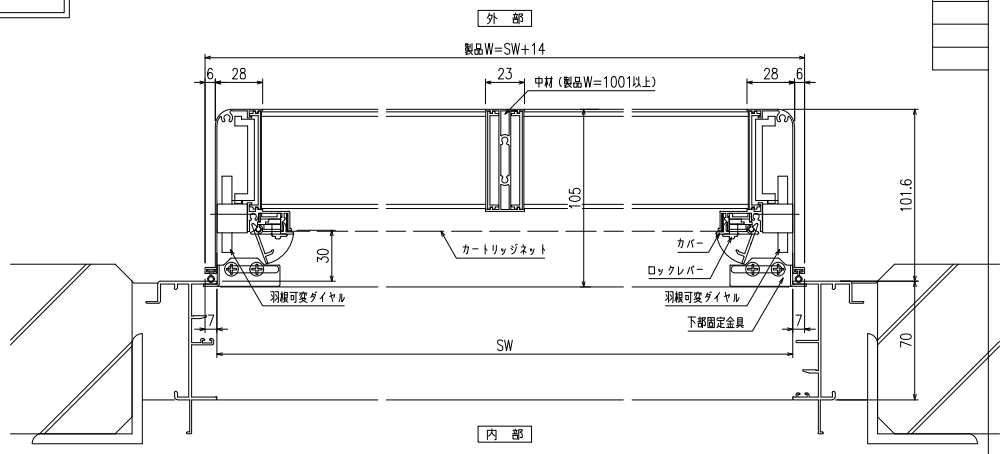
横断面図 (引き違い部分)
