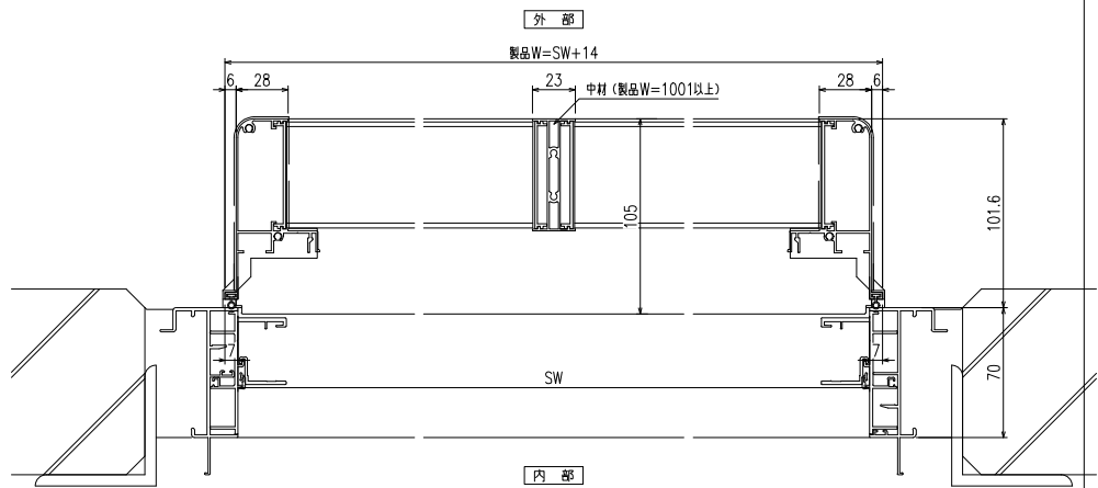
横断面図 (F1x部分)
