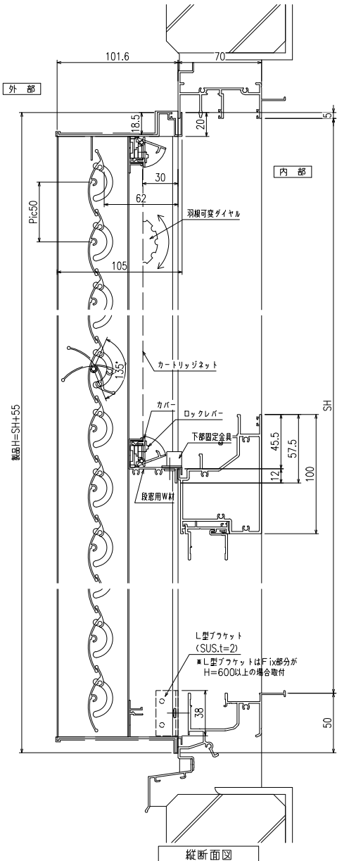
縦断面図
