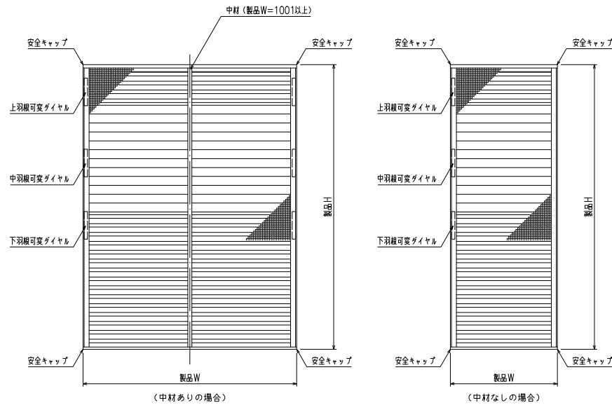
外観姿図
