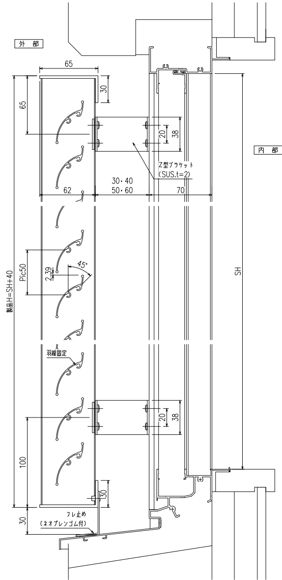
縦断面図
