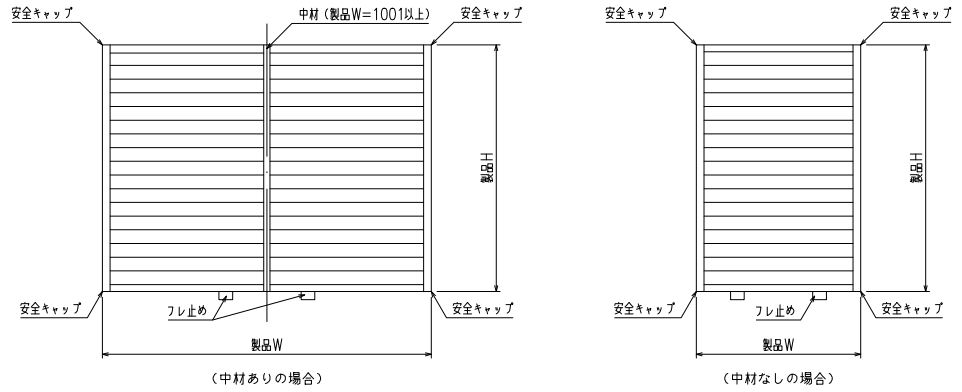
外觀姿図
