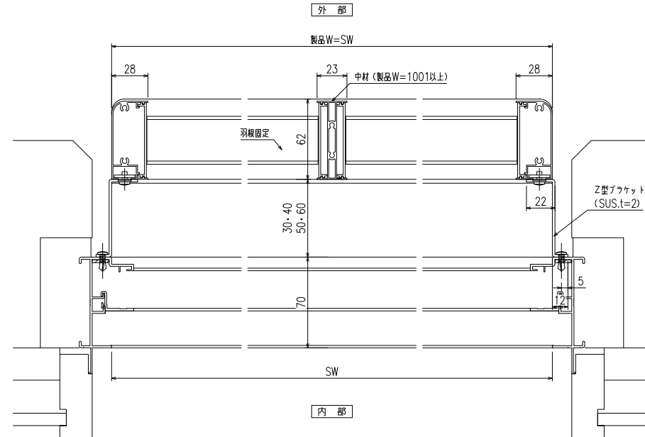
横断面図
