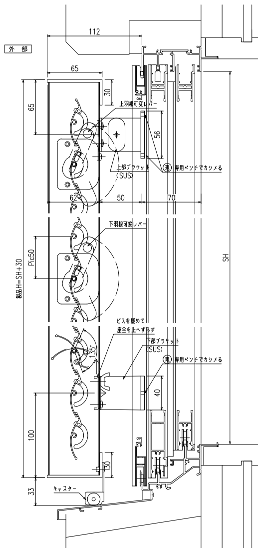
縦断面図
