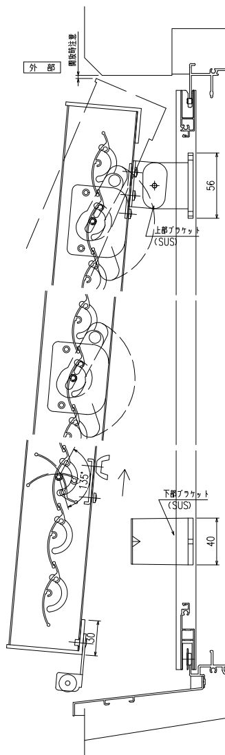
開放詳細図
