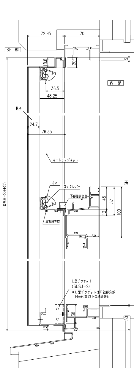
縦断面図
