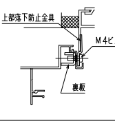
上部落下防止金具部分
