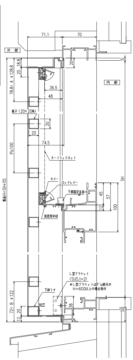
縦断面図
