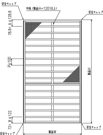
外觀姿図
