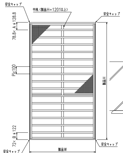
外觀姿図
