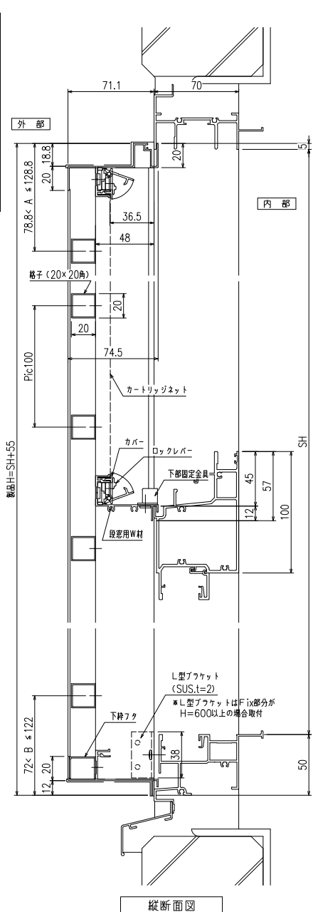
上部躯体のスキマ寸法について
