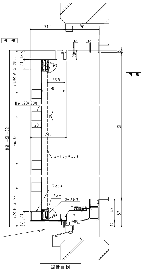
縦断面図
