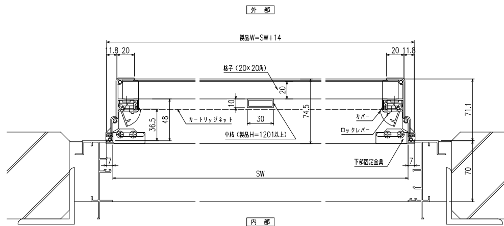
横断面図
