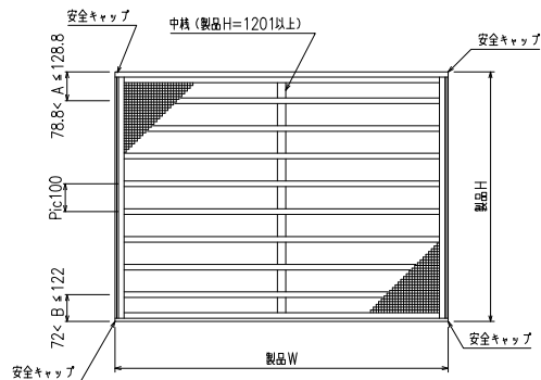
外観姿図
