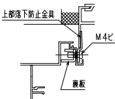
上部落下防止金具部分
