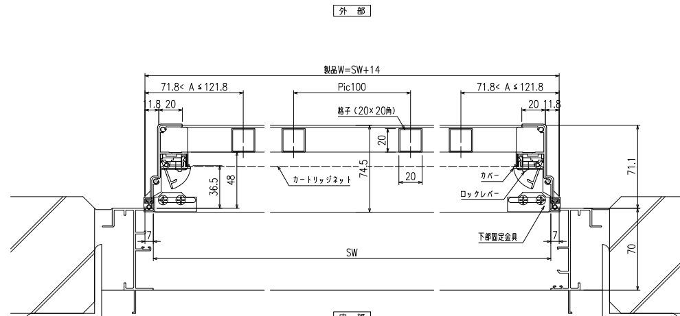
横断面図
