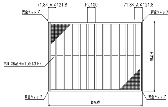
外観姿図
