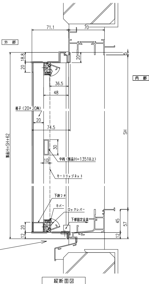
縦断面図
