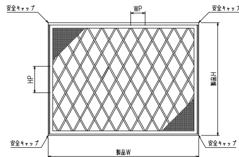
外観図
