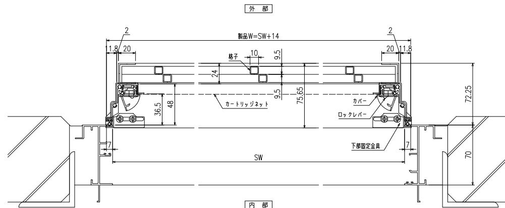
横断面図
