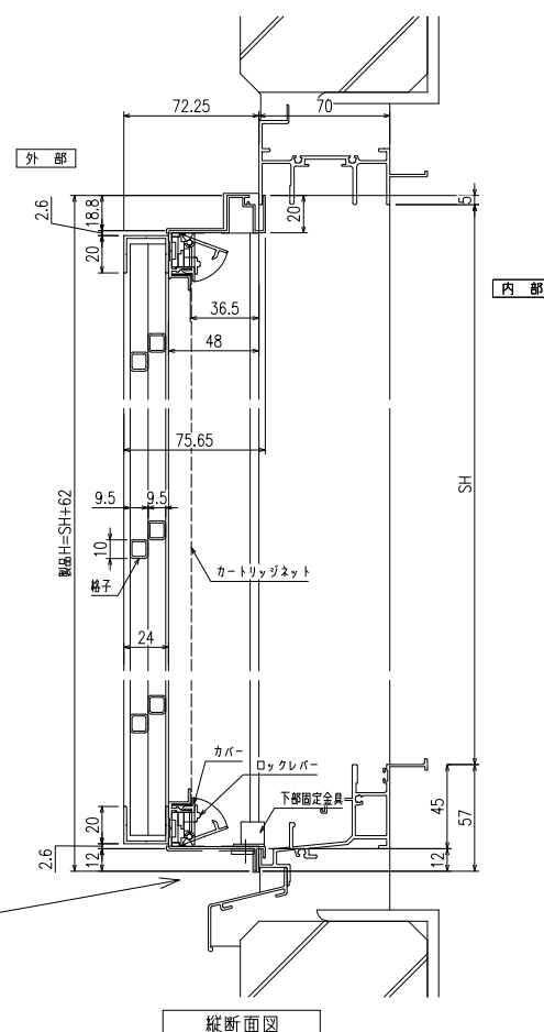
縦断面図
