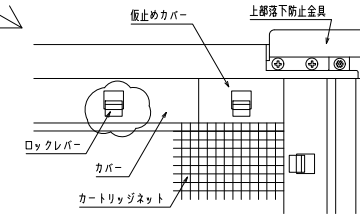
内観詳細図
