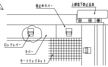
内観詳細図
