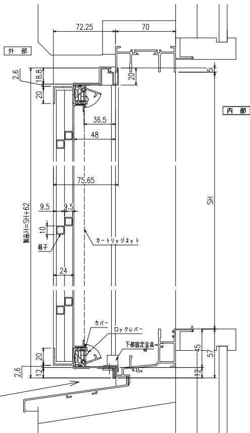
縦断面図
