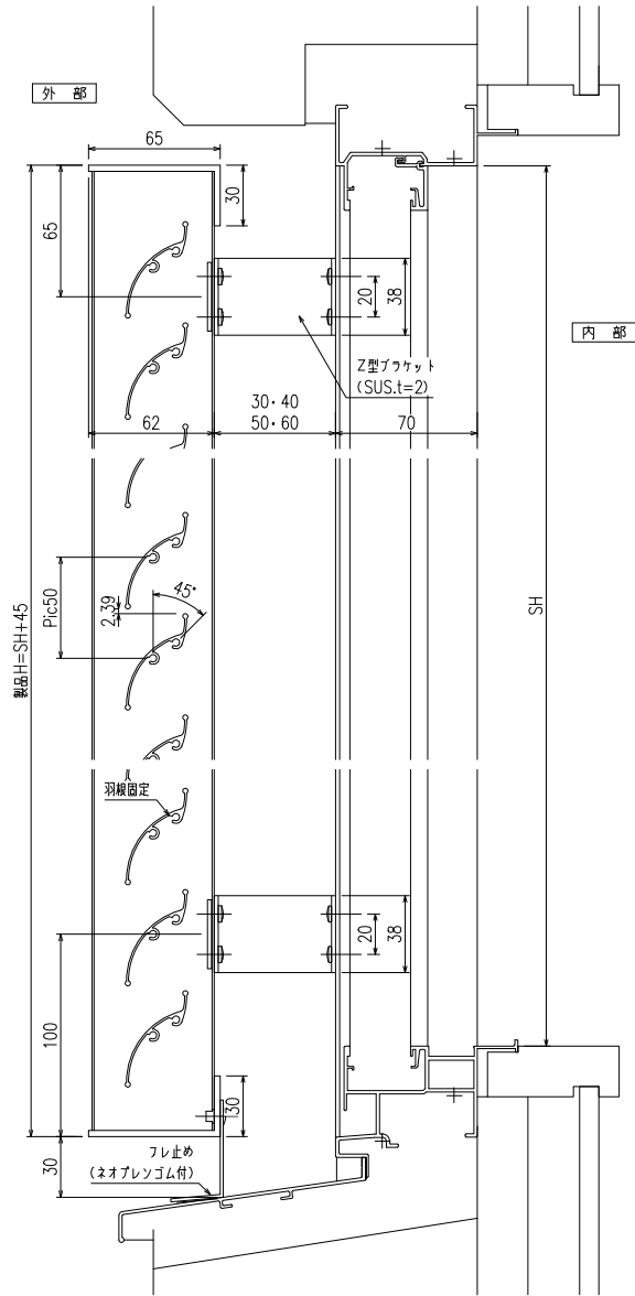
縦断面図
