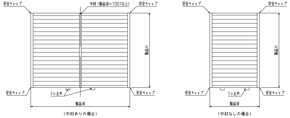
外観姿図
