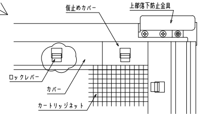
内観詳細図
