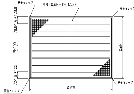
外観姿図
