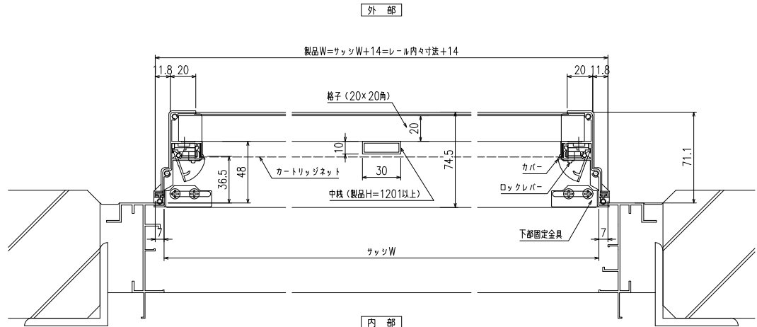
横断面図
