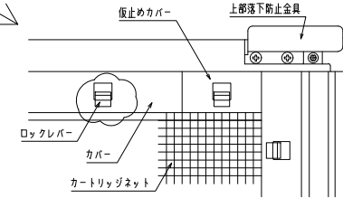
内観詳細図
