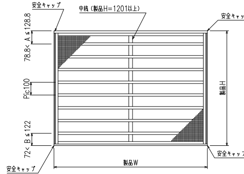
外觀姿図
