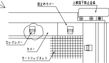
内観詳細図
