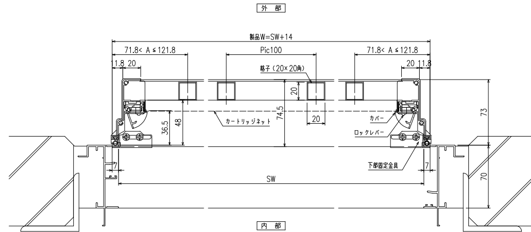
横断面図
