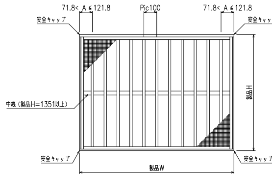
外觀姿図
