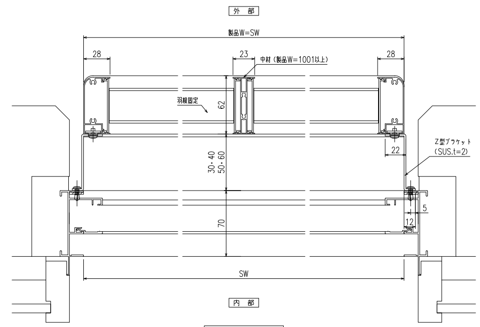
横断面図
