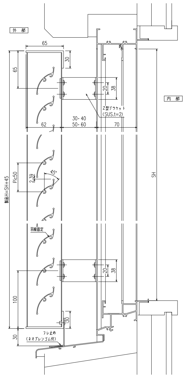
縦断面図
