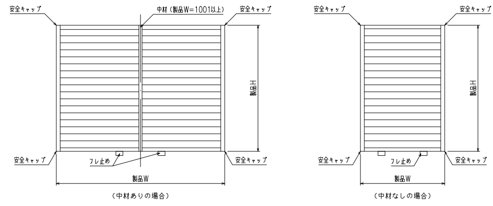
外觀姿図
