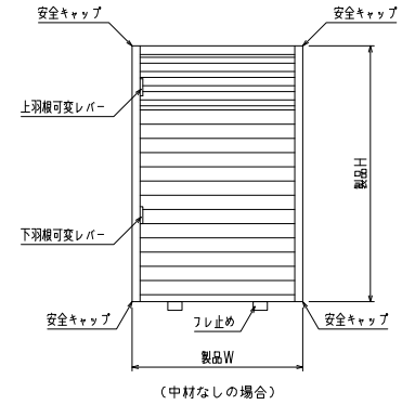
外観図
