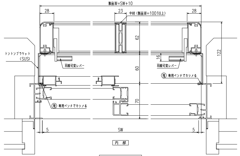
横断面図
