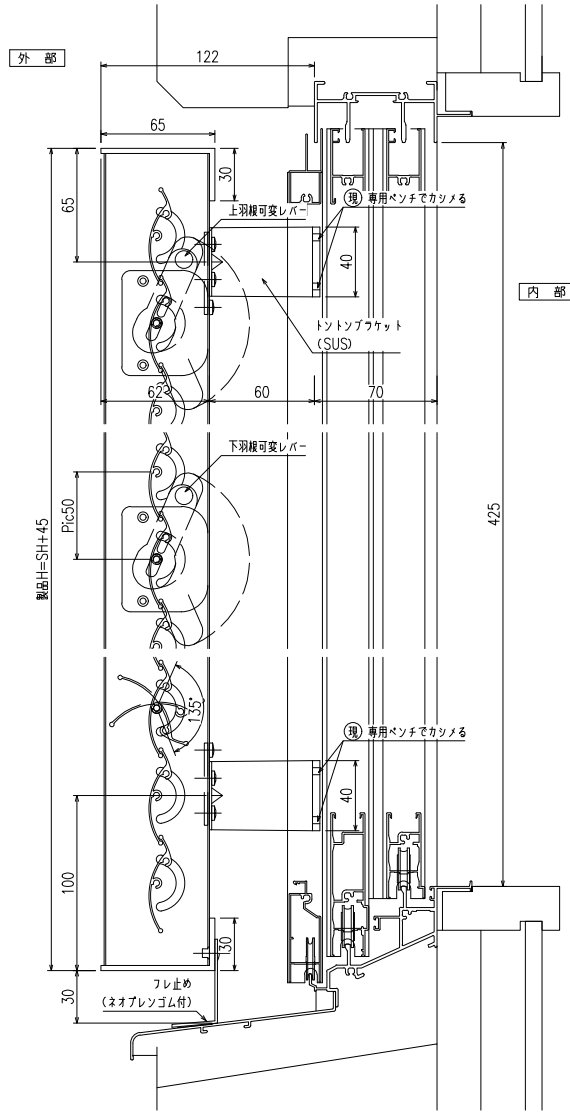
縦断面図
