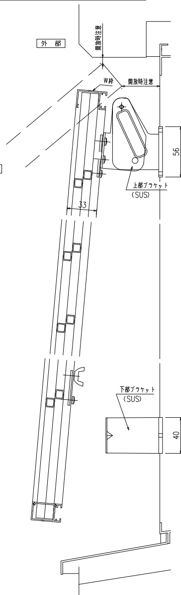
開放詳細図
