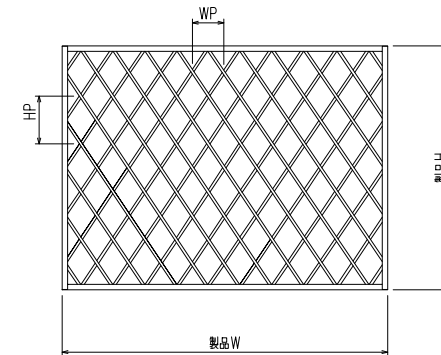
外觀姿図
