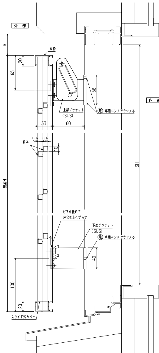
縦断面図
