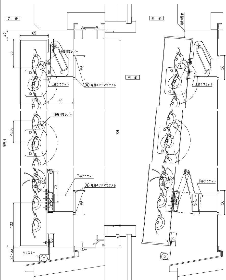
縦断面図
