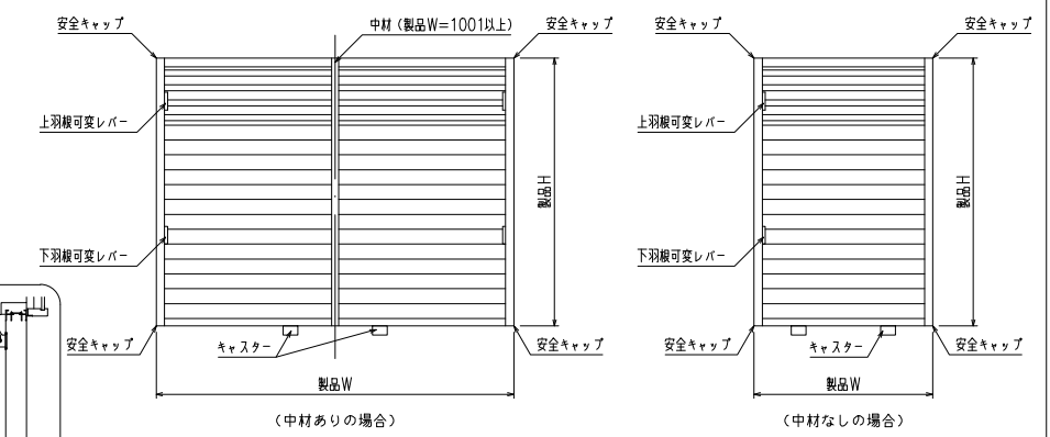
外観姿図
